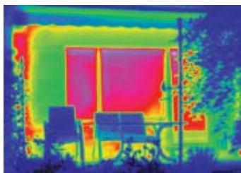
Les images de thermographie infrarouge permettent de visualiser les voies de déperdition de chaleur d'une maison. Le rouge représente la chaleur et par conséquent les pertes d'énergie.
